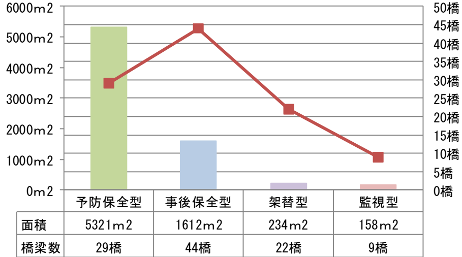
図 2-3-6 管理手法別橋面積比
